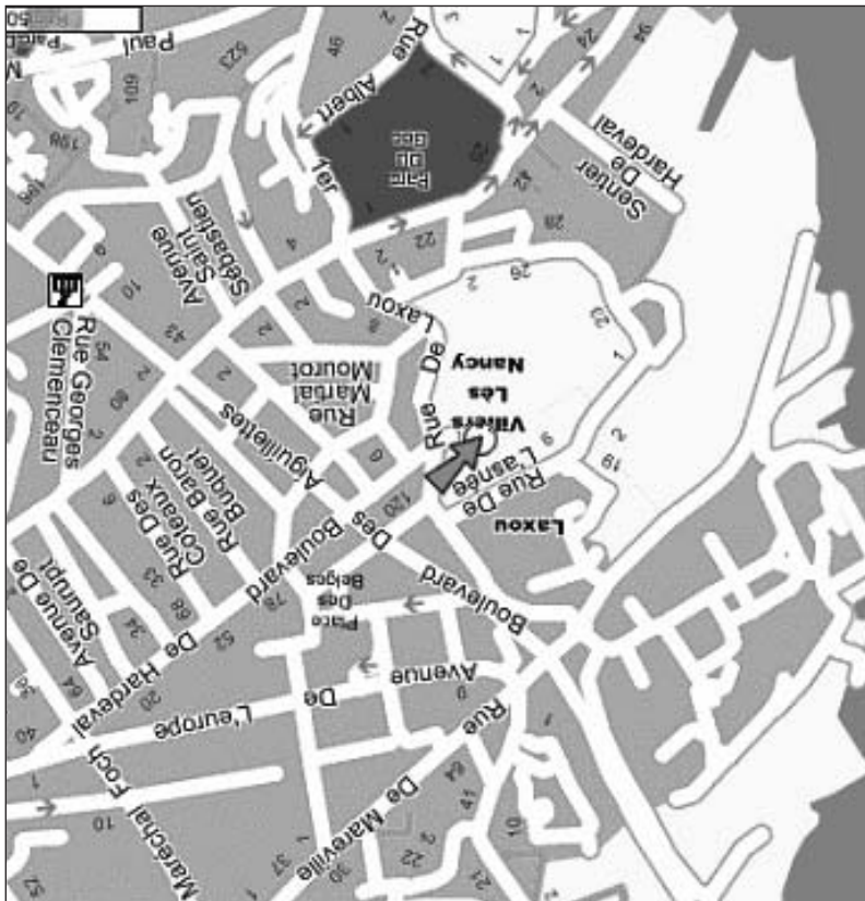
PLAN D'ACCÈS
